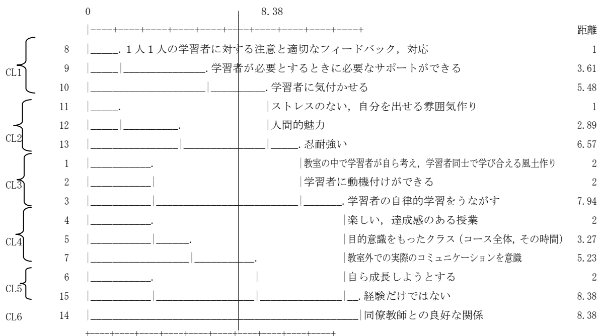
図1 教師Xのデンドログラム (7)
